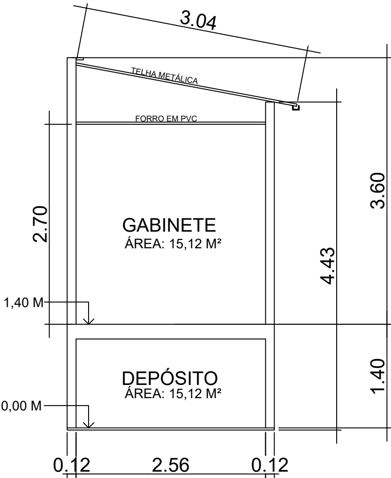
CORTE ESCALA.....1/50
